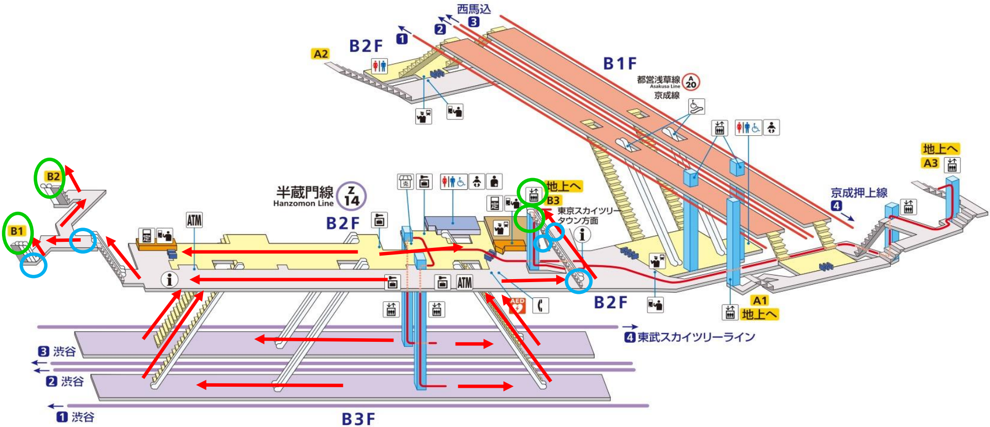
押上<スカイツリー前>駅構内立体図
