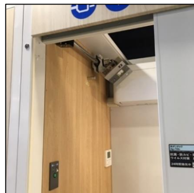
紫外線照射装置
